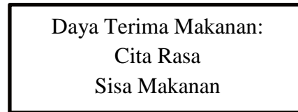
Gambar 1. Kerangka Konsep
