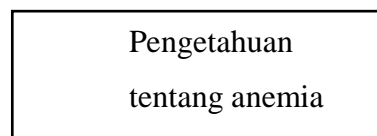
Gambar 2. Kerangka Konsep
