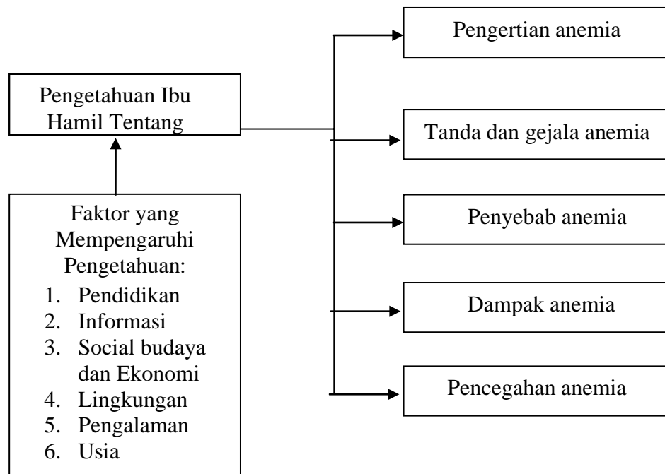
Gambar 1. Kerangka Teori
